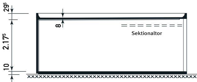
Schnitt
