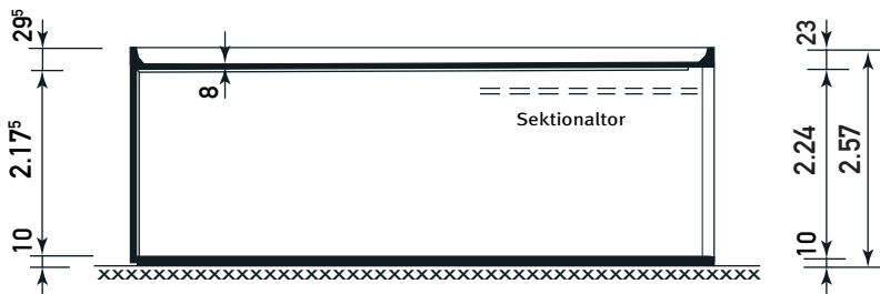
Schnitt
