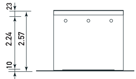
Rückansicht
