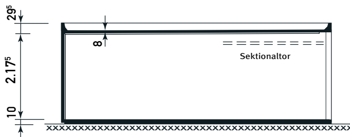
Schnitt
