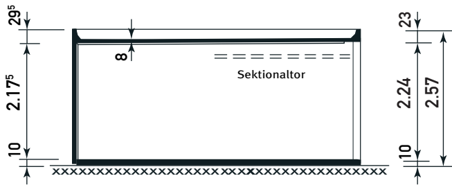
Schnitt
