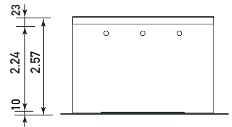
Rückansicht
