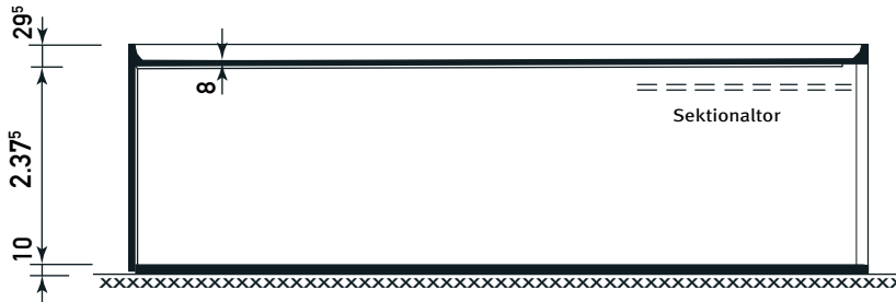
Schnitt
