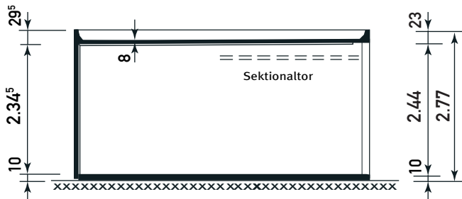
Schnitt
