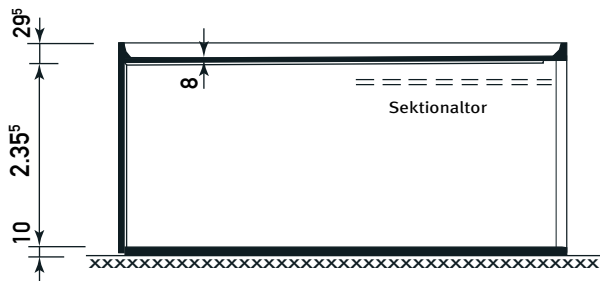
Schnitt
