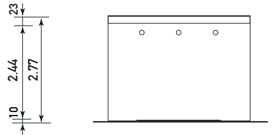
Rückansicht
