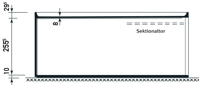
Schnitt
