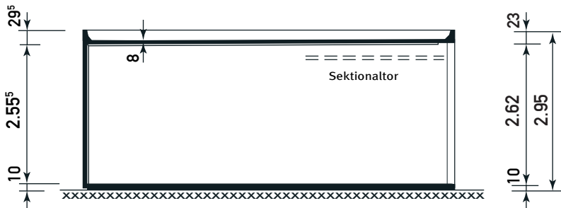
Schnitt
