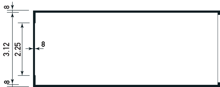
Grundriss
