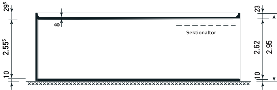
Schnitt
