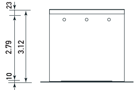
Rückansicht
