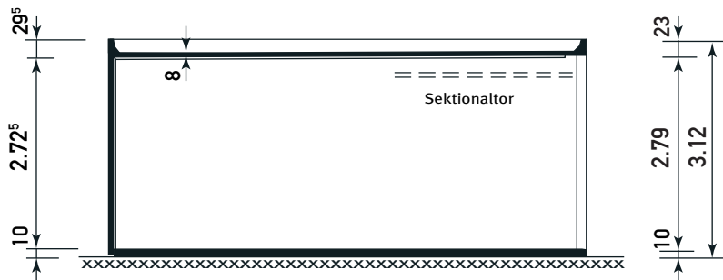
Schnitt
