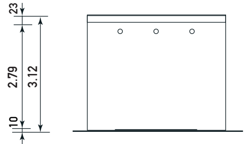
Rückansicht
