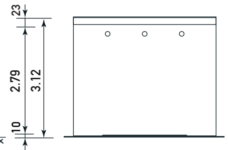
Rückansicht
