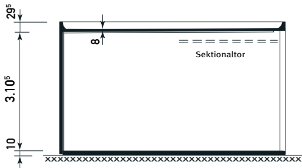
Schnitt
