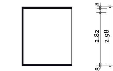
Grundriss
