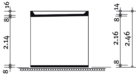
Schnitt
