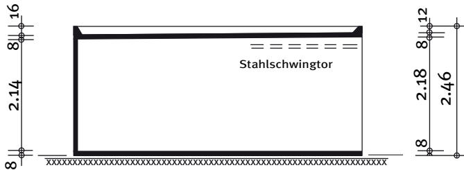
Schnitt
