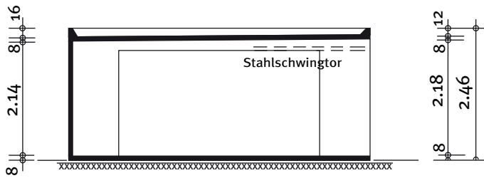
Schnitt
