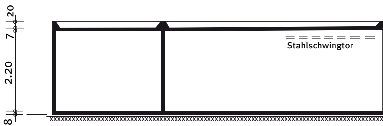
Schnitt
