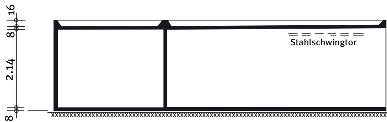
Schnitt
