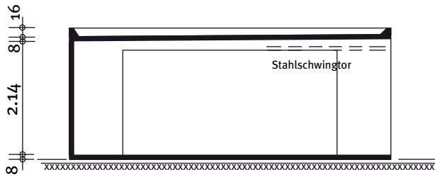
Schnitt
