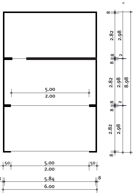
Grundriss
