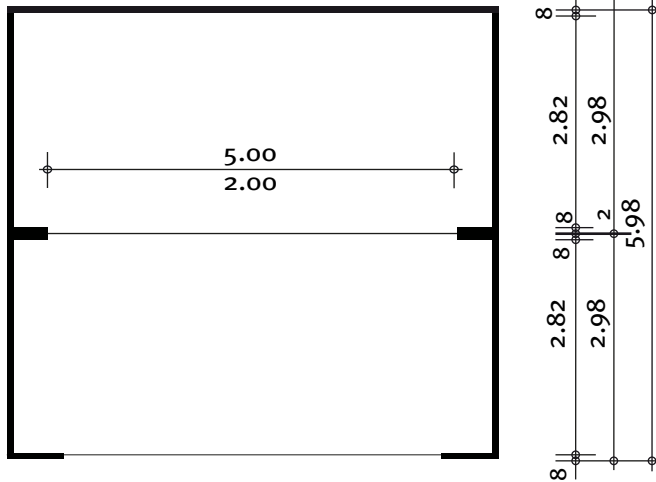
Querschnitt
