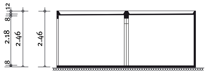
Längsschnitt
