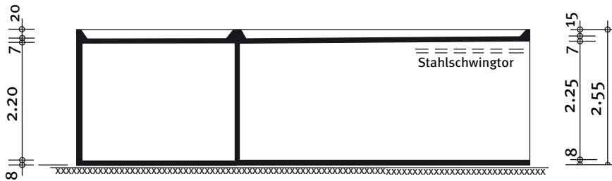
Schnitt
