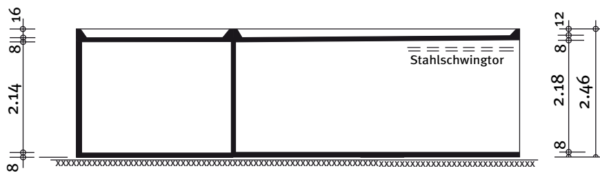
Schnitt
