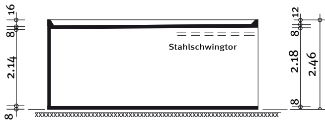
Schnitt
