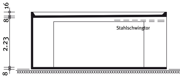
Schnitt
