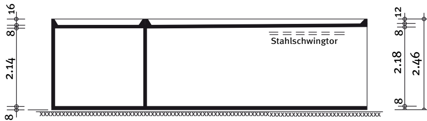
Schnitt
