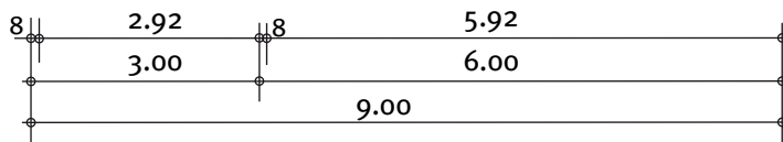
Grundriss
