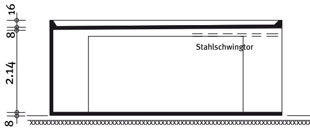
Schnitt
