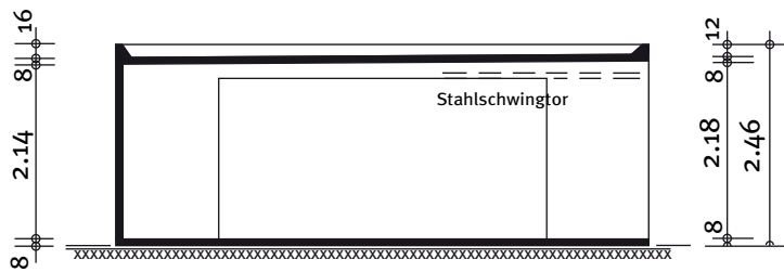
Schnitt
