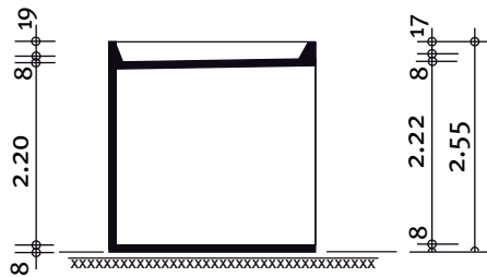
Schnitt
