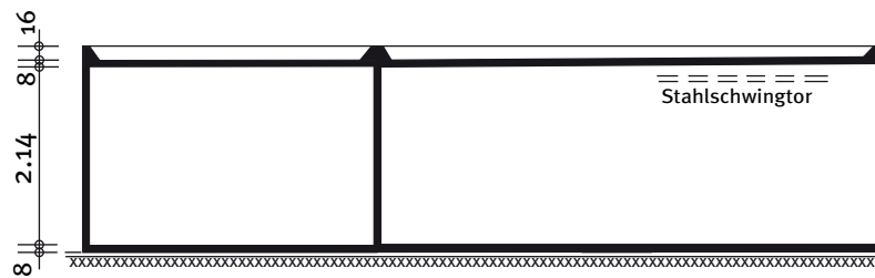
Schnitt
