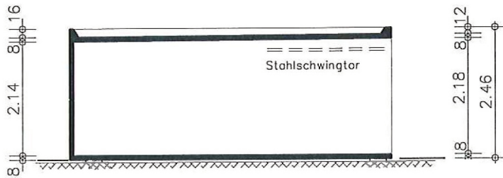
Schnitt
