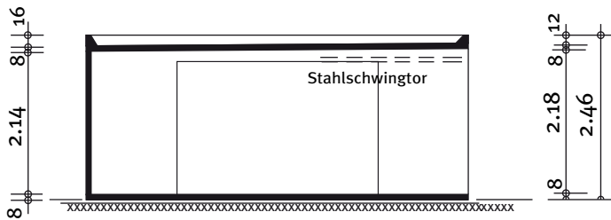
Schnitt
