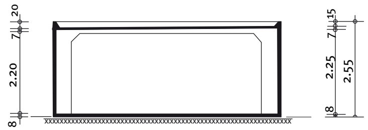
Schnitt
