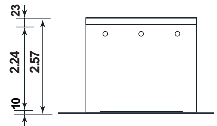
Rückansicht
