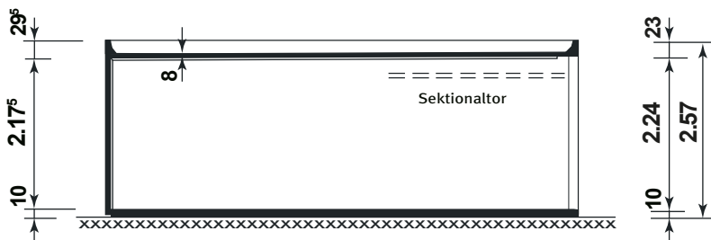
Schnitt
