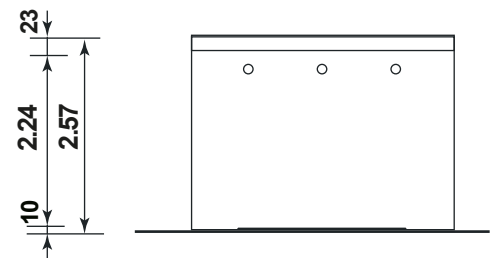
Rückansicht
