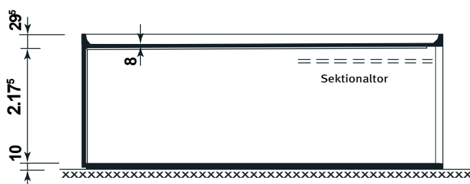
Schnitt
