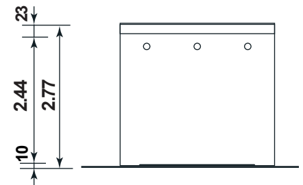
Rückansicht
