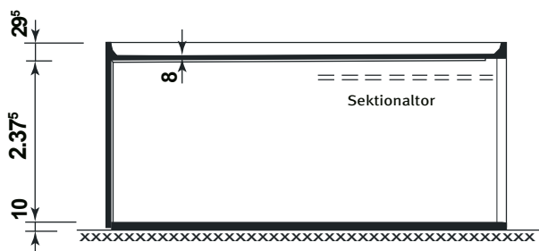
Schnitt
