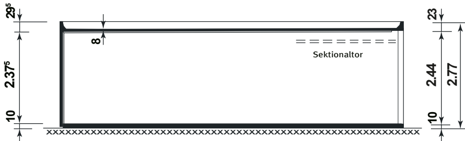
Schnitt
