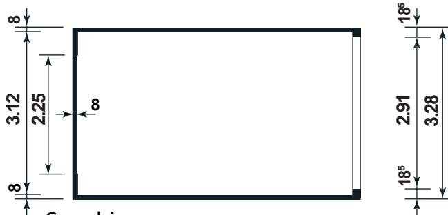
Grundriss
