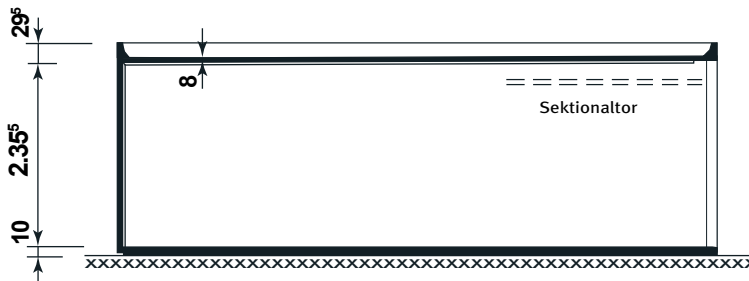
Schnitt
